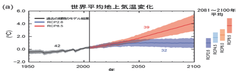
図A 世界平均地上気温の変化(1986～2005年平均からの偏差) 予測と不確実性の幅(陰影)の時系列を、RCP2.6とRCP8.5のシナリオについて示した。 出典 気候変動に関する政府間パネル第5次評価報告書 第1作業部会報告書 気候変動2013:自然科学的根拠 政策決定者向け要約 気象庁訳(2015年12月1日版) http://www.data.jma.go.jp/cpdinfo/ipcc/ar5/ipcc_ar5_wg1_spm_jpn.pdf
