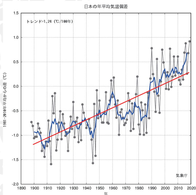
図1 日本の年平均気温偏差 細線黒丸：各年の平均気温の基準値からの偏差，太線：偏差の5年移動平均値，直線：長期変化傾向。基準値は1981～2010年の30年平均値。
